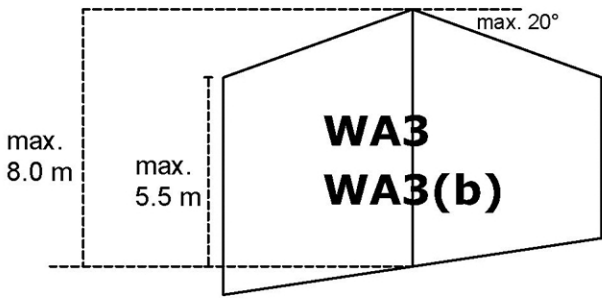
Zeltdach / Satteldach
